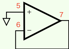
未使用オペアンプ
