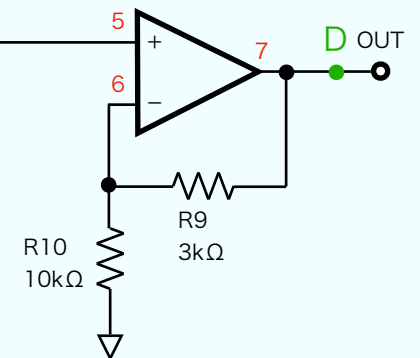
出力回路
