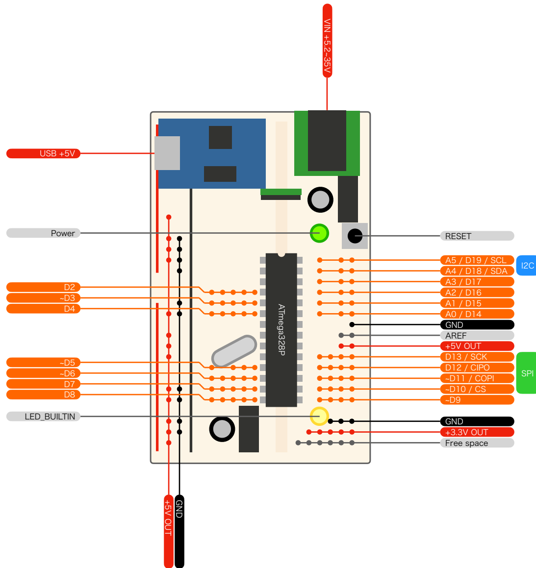
ATmega328Pマイコンボード ピン配置図
