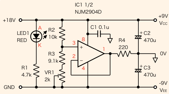
電源回路
